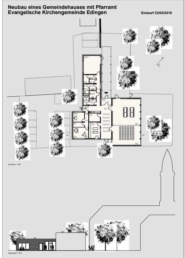
Grundriss mit Aufteilung in großen Saal, der keine Trennwand enthalten soll, Foyer, Küche, Pfarramt, Sanitärräume und Jugend- bzw. Mehrzweckraum.
